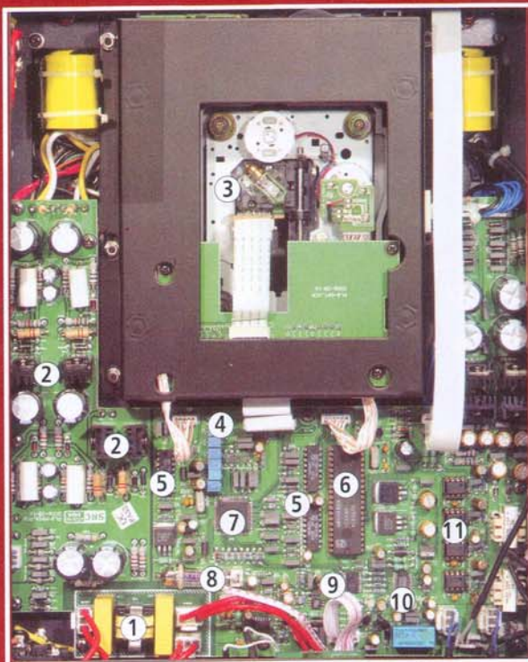
Vue interne 1 - Filtrage du secteur par circuit en « PI ». 2 - Après redressement par les tubes 5AR4 situés sur le dessus de l'appareil, les alimentations sont filtrées puis stabilisées à l'aide de 11 régulateurs distincts accompagnés de composants de premier choix (résistances de précision, condensateurs Solen, etc.). 3 - Base mécanique avec bloc optique Sony KSS 213 Q. 4 - Etage « servo », gestion des asservissements. 5 - Circuits drivers de puissance TDA 7073 (mécanismes d'asservissements). 6 - Microcontrôleur 8 bits de gestion OM4368BN (équivalent à P89C58). 7 - Processeur « servo » numérique SAA 7327. 8 - Système d'horloge inédit « SuperTubeClock ». Il utilise un tube triode subminiature dont la fréquence d'oscillation sinusoïdale est convertie en signal carré. La précision de ce circuit est extrême, avec un signal carré d'une fréquence de plus de 8 MHz présentant des fronts de montée et de descente parfaitement réguliers et ultra-rapides. Cet oscillateur est utilisé pour la section Drive (cadence des datas) et la section DAC (resynchronisation). Il est réalisé autour d'un tube 656B-V « spécification militaire » d'origine russe. 9 - Circuit Burr-Brown SRC 4192 utilisé pour reformater le signal numérique en 24/192 kHz. 10 - Convertisseur Burr Brown PCM 1792, 24 bits / 192 kHz. 11 - Conversion courant - tension par quatre amplis opérationnels NE5532 (configuration symétrique).
